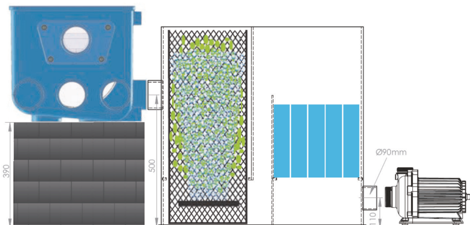
SBSG560 Bio Kammer mit bewegenden-Filtermedien Modul inkl. Eco-Pond-Chips und T-Profil Filterschaummatten
