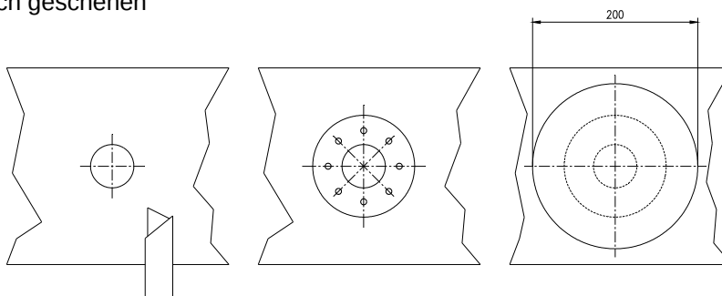
Abbildung: Nachträgliche Montage Mauerdurchführung bei Folienbecken
