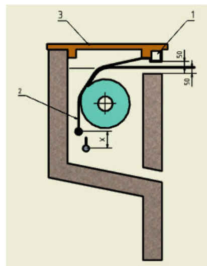
Abbildung z.B. Sturzbalken im Rucksackschacht montieren
