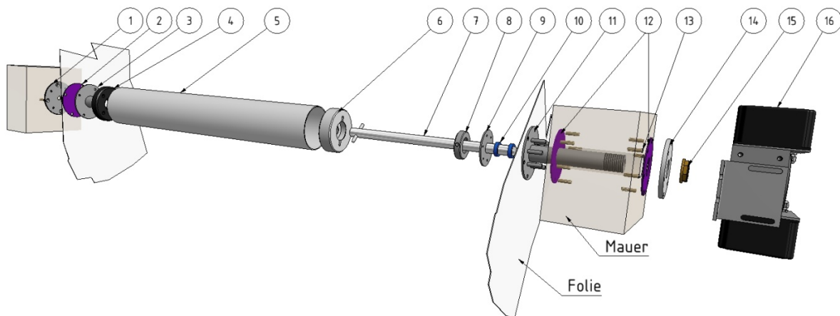
Abbildung: Explosionszeichnung Aufrollvorrichtung
