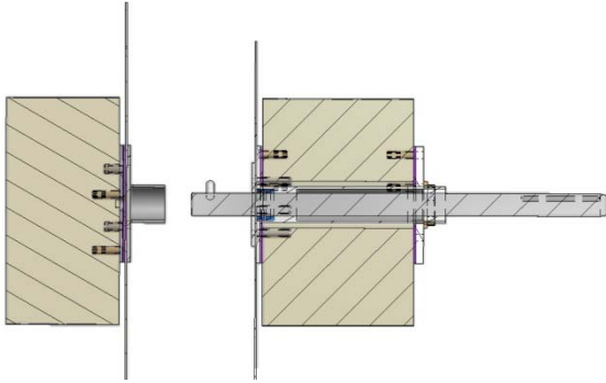
Abbildung: Montage Folienbecken
