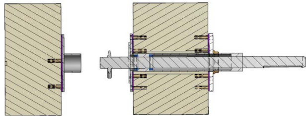
Abbildung : Montage Betonbecken
