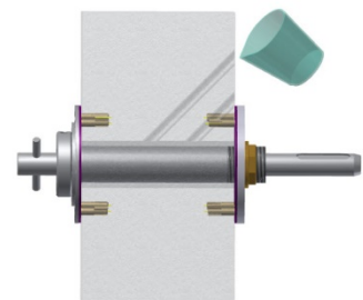
Abbildung: Schemazeichnung Mauerdurchführung vergiessen
