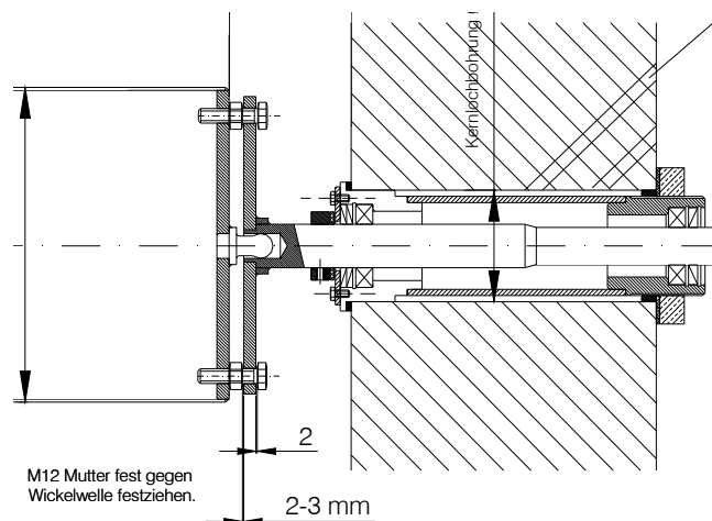
Abbildung 7: Einstellen der Antriebswelle
