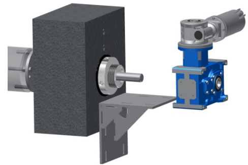
Abbildung 8: Montage Antrieb
