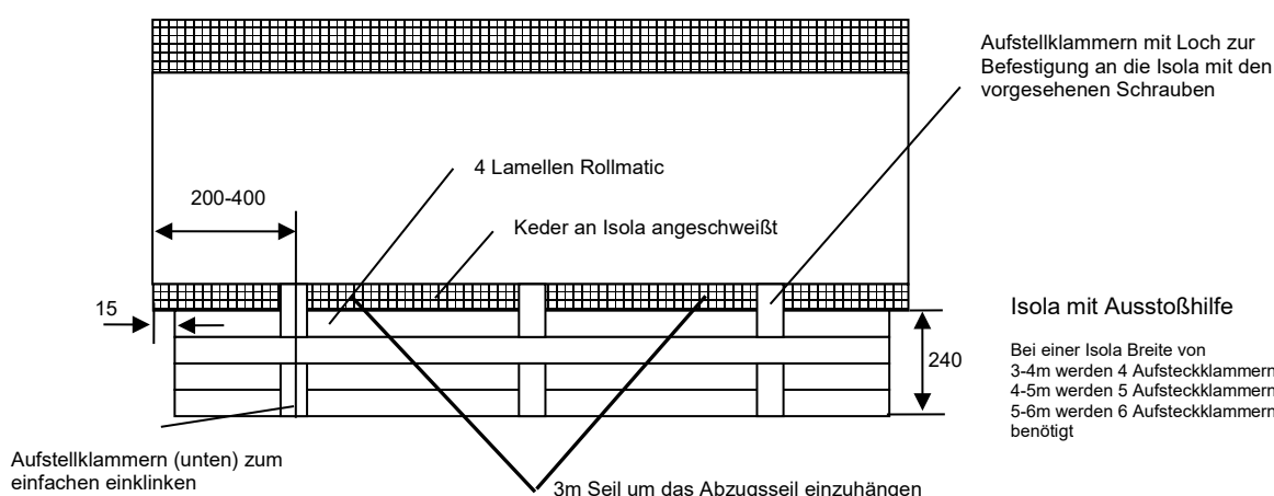
Skizze Isola mit Ausstosshilfe
