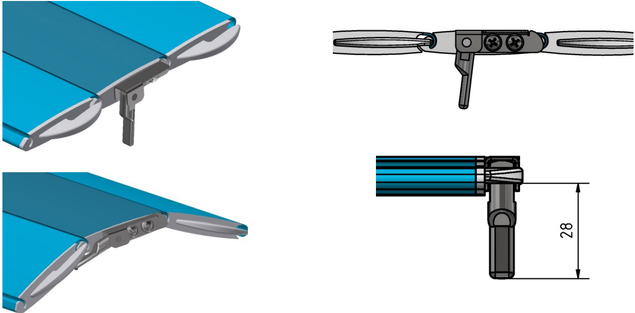
Abbildung 2-7: Abweiser
