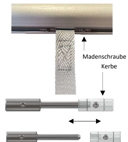
Abbildung 3-1: Einhängestift lösen
