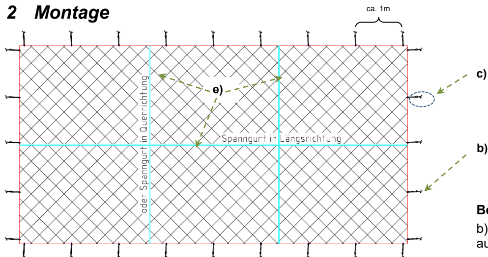
Abbildung 2.1: Beispiel Schutznetz-Montage
