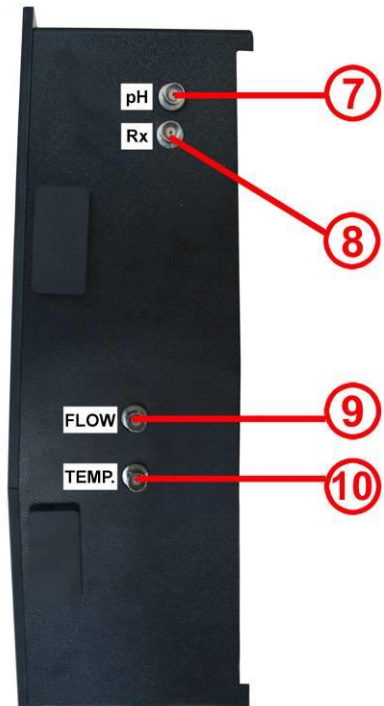
Bild: Reglergehäuse von rechts
