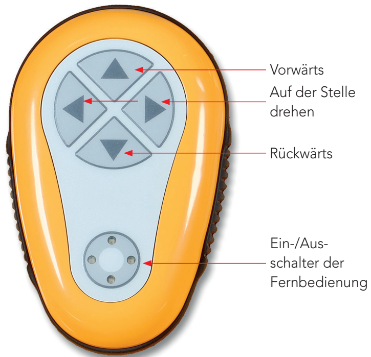
Abbildung 16: Fernbedienungseinheit
