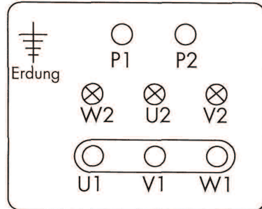
Pumpenschaltkasten 400 V
