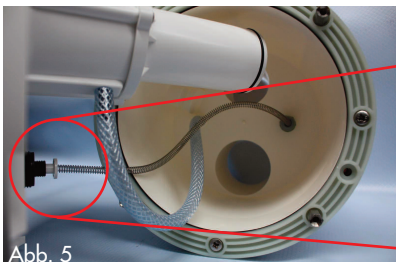
Abb. 5 Betriebsanleitung Gegenstromanlage ST 800 / ST 900 / ST 1050 / ST 1150 V.20150327
